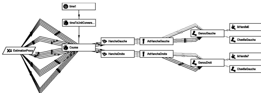
FIG. 16 – Sous-graphe associé à la synthèse du mouvement de course, mixant des modèles dynamiques et cinématiques (un sous-graphe similaire est associé à la jambe droite).
