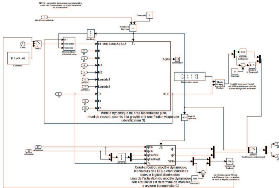
FIG. 17 – Modèle dynamique, échantillonné, de bras créé avec Simulink.
