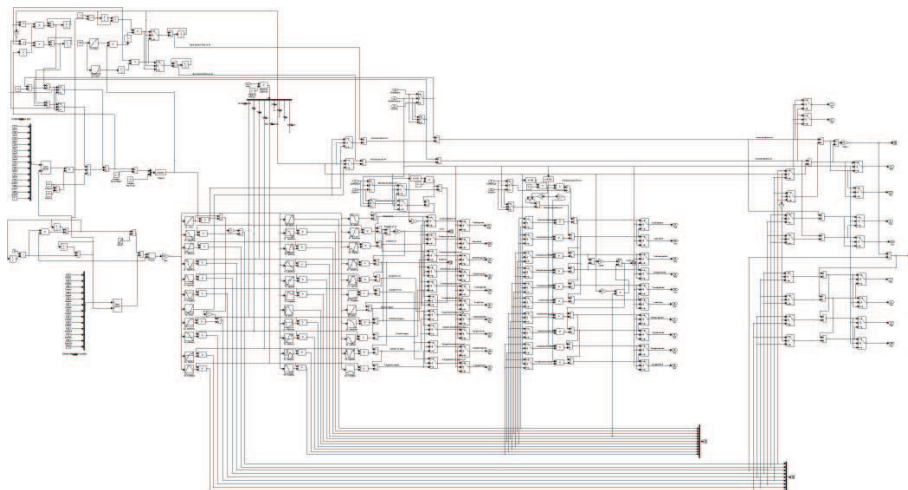
FIG. 18 – Modèle procédural de course créé avec Simulink.
