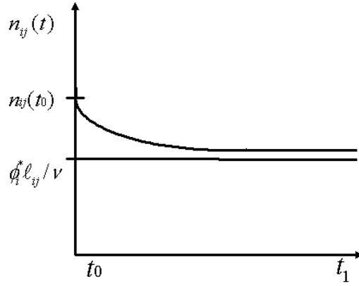
Figure 2: Evolution of n_{ij}(t) when n_{ij}(t_0) > \phi_i^* l_{ij} / \nu
