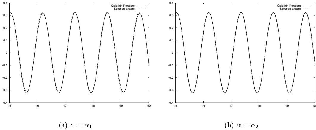
FIG. 12 – Composante E_z : évolution en temps / Raffinement 1:4 / Maillage : \lambda/8
