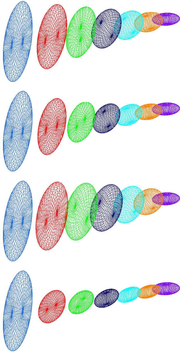
FIG. 6 – Comparaison des divers schémas d'interpolation en dimension trois. De haut en bas on a, le schéma linéaire (1), le schéma géométrique (2), le schéma linéaire en \mathcal{M}^{-1} (3) et l'interpolation termes à termes. Dans le contexte de l'adaptation de maillages, on préférera l'un des trois premiers schémas pour l'interpolation de métriques.
