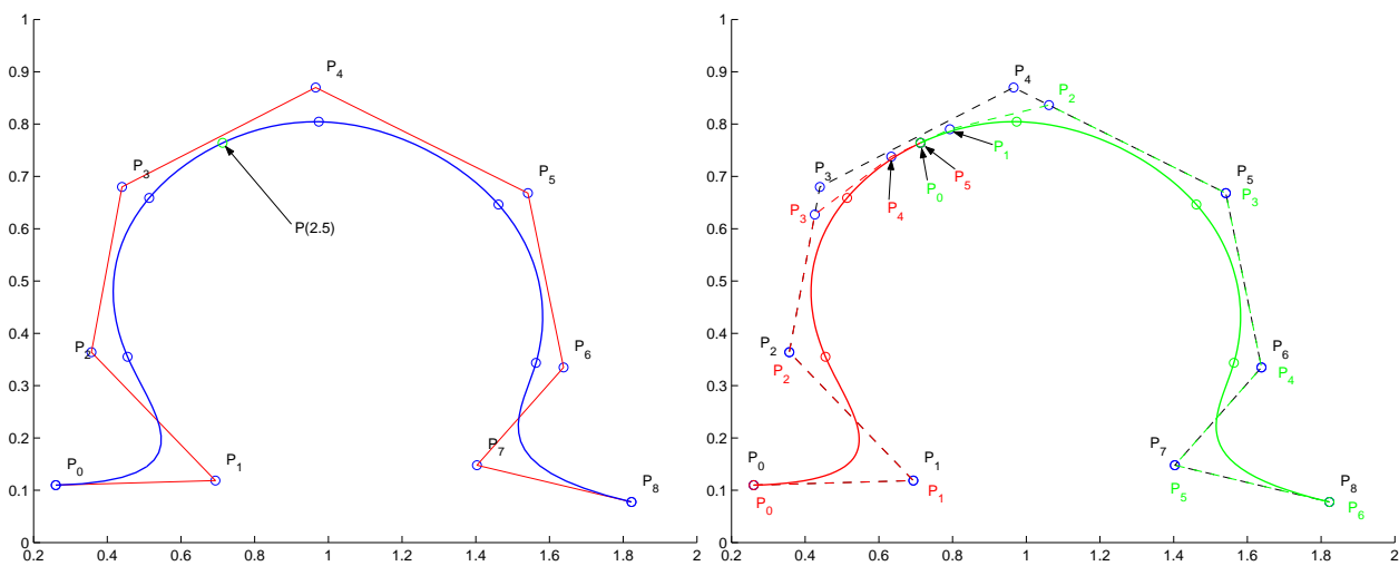
FIG. 6 – Courbe B-spline pour le vecteur nodal [0,0,0,0,1,2,3,4,5,6,6,6,6] (courbe initiale à gauche et subdivision en u = 2.5 à droite) RR n° 4968
