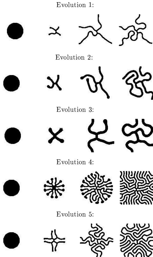
FIG. 1.6 – Évolutions géométriques pour différentes valeurs des paramètres d_{min} (trois premières lignes) et \alpha (deux dernières lignes).
