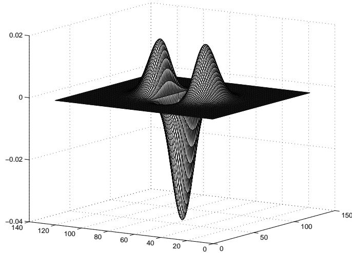
FIG. 2.4 – Filtre utilisé pour la construction de la carte ( \sigma_x = 4 , \sigma_y = 1 ).
