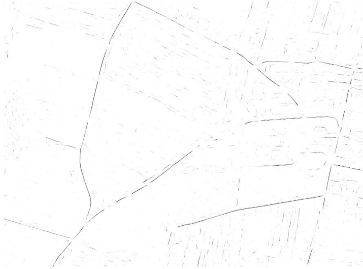
FIG. 2.8 – Carte de champ calculée avec les t-tests.
