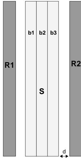
FIG. 2.5 – Masque pour les tests de Student.
