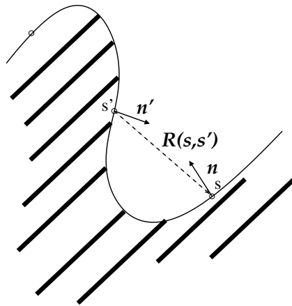
FIG. 1.4 – La fonction de pondération.
