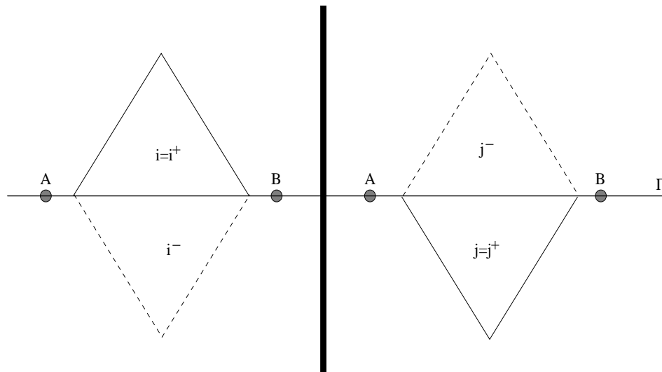
FIG. 3.5 – Deux cellules voisines de part et d'autre de la faille : contact parfait
