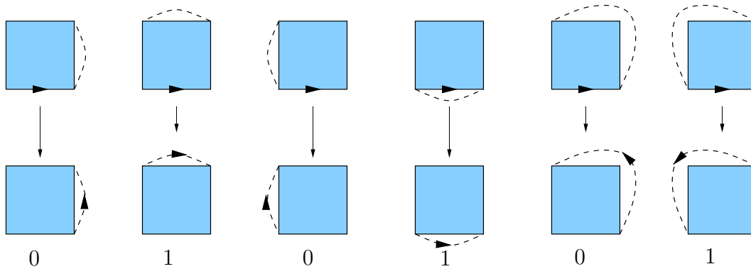
FIGURE 24. Règle d'attribution de l'orientation de la racine et du paramètre binaire.
