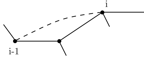
FIGURE 18. Création d'une arête entre un sommet i et un sommet i - 1 .
