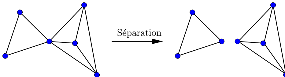
FIGURE 3. Une carte séparable.
