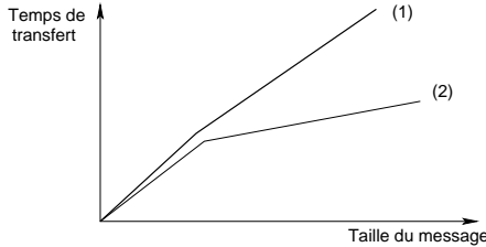
FIG. 9 – Allure de la courbe de transfert de données par copie en réception (1) à partir de l'allure de la courbe de transfert de données interne (2) (fig. 3). FIG. 10 – Allure de la courbe de transfert de données par rendez-vous en réception (1) à partir de l'allure de la courbe de transfert de données interne (2) (fig. 3).
