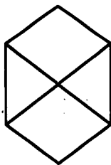
\neg \text{cpo}_\wedge
