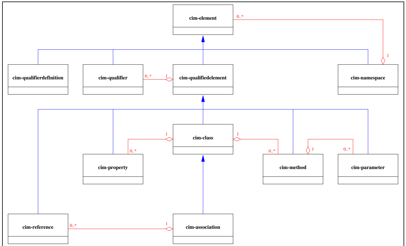
FIG. 5 – Les classes du schéma LDAP
