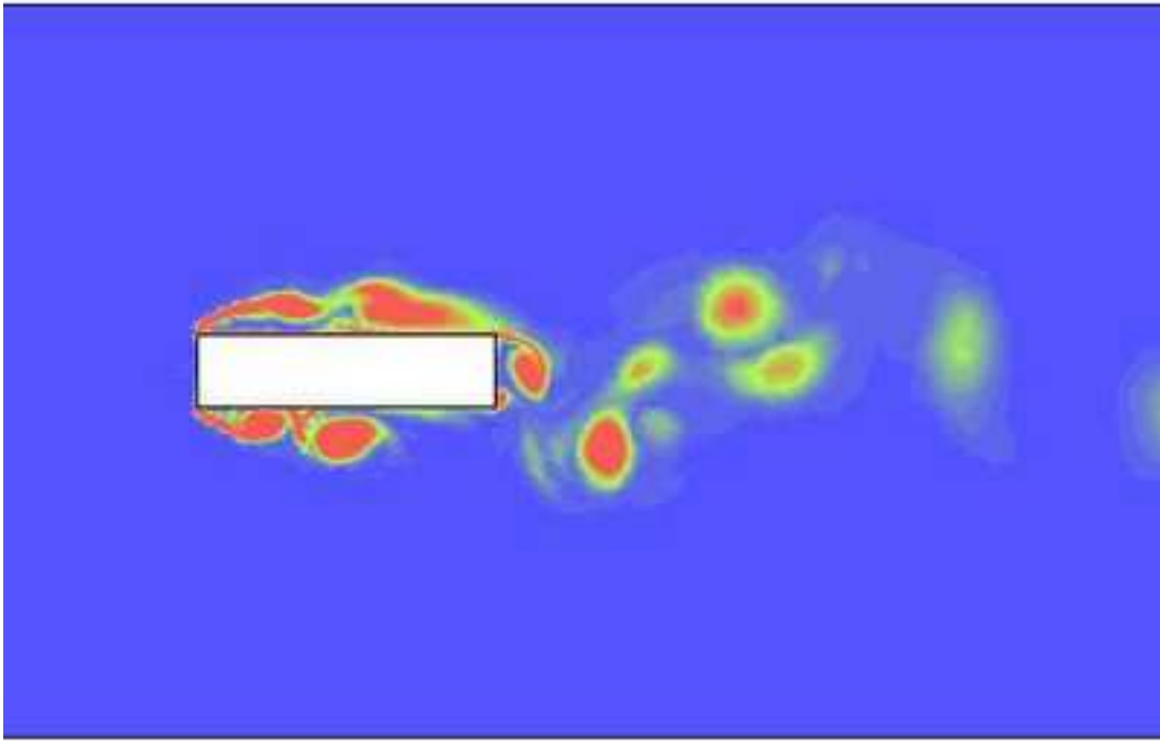
FIG. 40 – Vorticité autour du profil.
