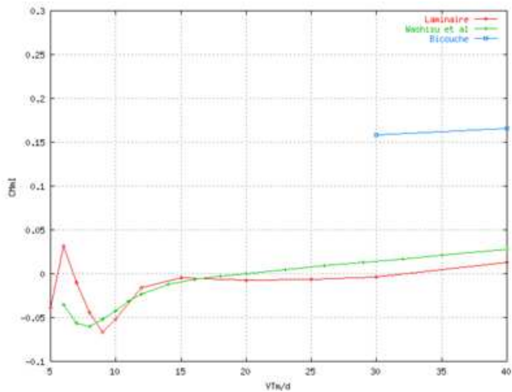
FIG. 46 – CMmI en fonction de la période du forge
