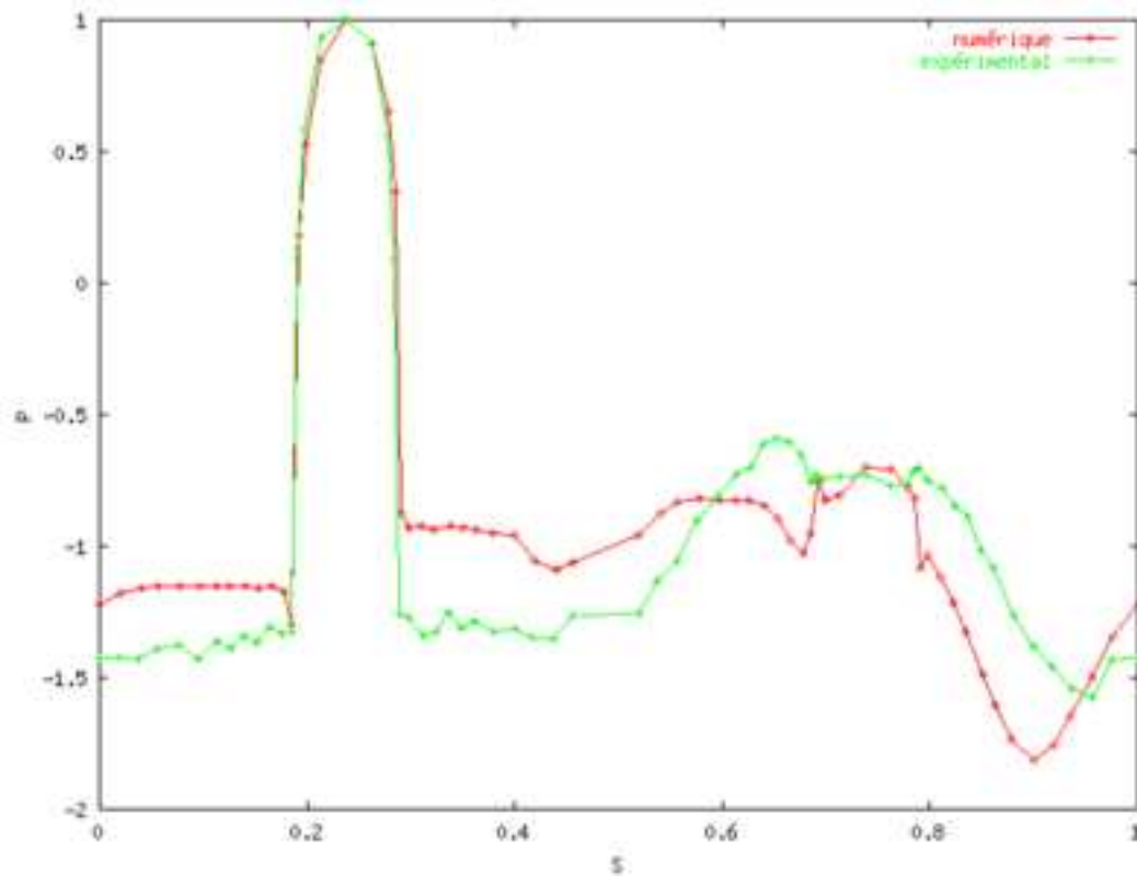
FIG. 36 – Profil de pression
