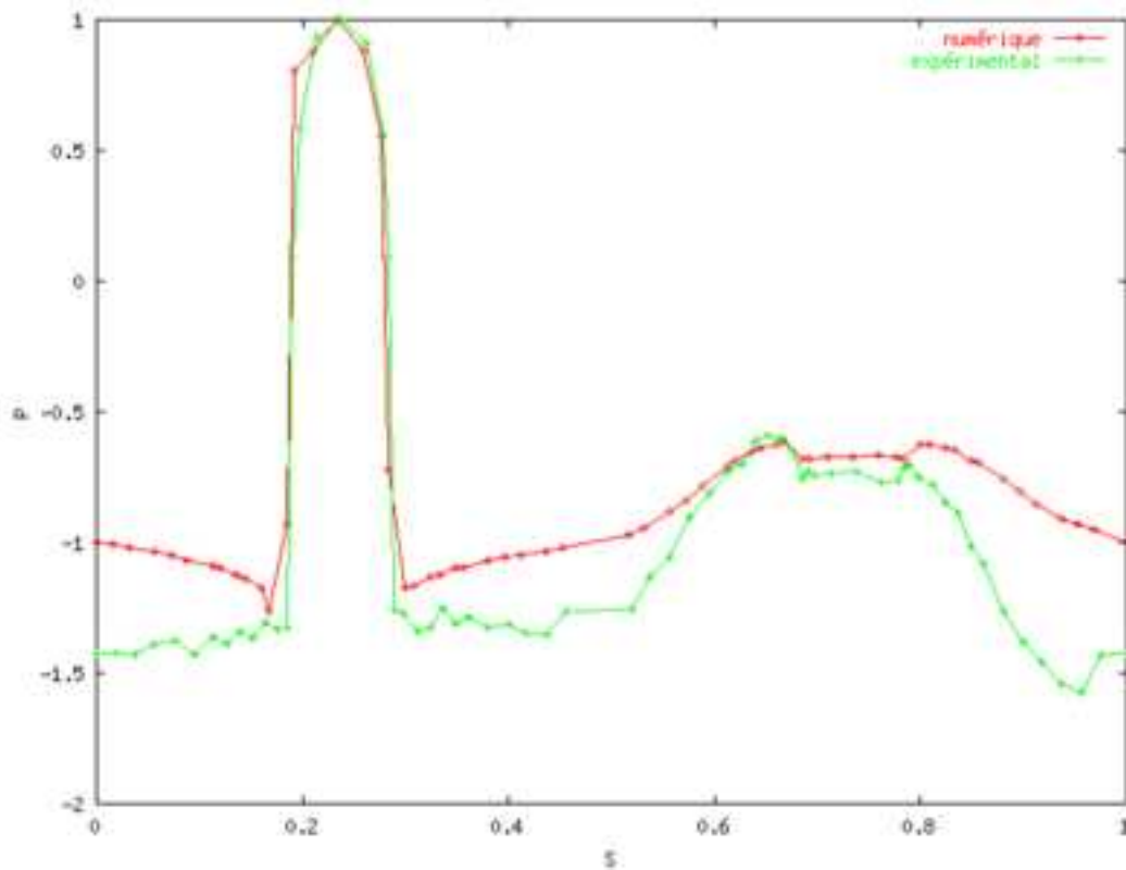
FIG. 7 – Profil de pression
