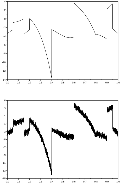
FIG. 2 - Signal polynomial par morceaux, et avec bruit \text{SNR} = 21.9 dB.
