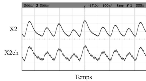
FIG. 8 – Reconstruction de x_2 ; en haut : x_2 , en bas : \hat{x}_2
