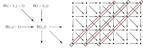
FIG. 11 – Localité du calcul dans une cellule SW/NW (à gauche). Les flèches noires montrent les scores provenant des trois cellules précédentes. La seule autre information dont la cellule a besoin est d(x_i, y_j) . Les flèches en pointillés montrent la propagation des données vers les trois cellules suivantes. Lorsqu’on cherche à calculer toutes les cellules d’une matrice de programmation dynamique, les cellules le long d’une même anti-diagonale peuvent être calculées simultanément (à droite).
