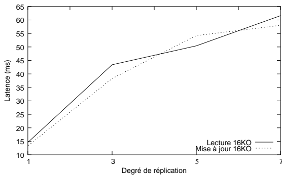
FIG. 4 – Performance des accès sur une donnée de 16 KO selon le degré de réplification.
