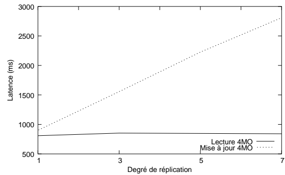
FIG. 5 – Performance des accès sur une donnée de 4 MO selon le degré de réplification.
