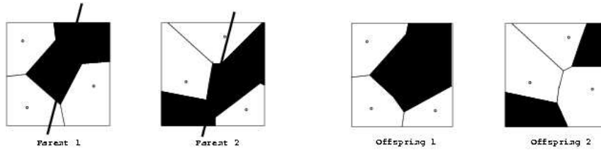
FIG. 2 – La représentation de Voronoï et ses opérateurs de croisement : une droite aléatoire est tracée dans chaque diagramme et les sites sont échangés d’un côté de cette droite
