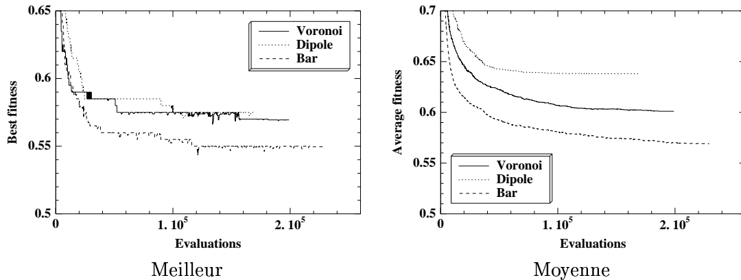
FIG. 12 – Représentations de Voronoï sur le cantilever 2 \times 1 pour D_{lim} = 220 .
