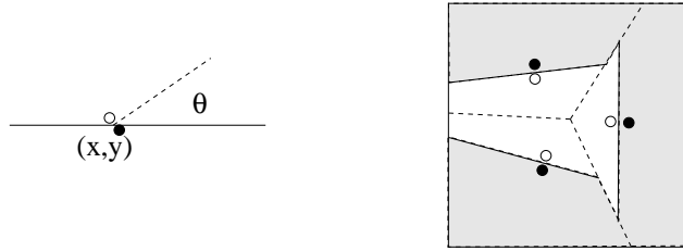
FIG. 3 – La représentation par dipôles. Un seul dipôle (a) et le diagramme de Voronoï construit à l’aide de trois dipôles (b) : des coins indésirables apparaissent aux croisements des médianes.
