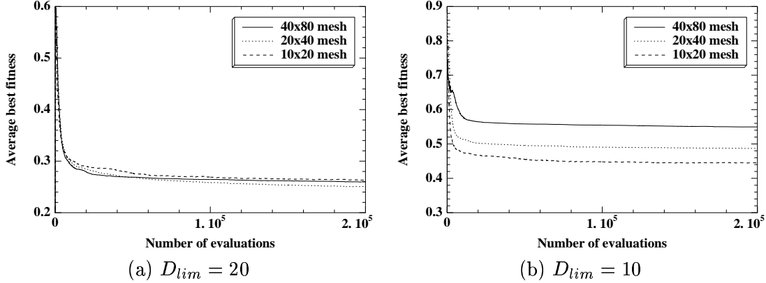
FIG. 5 – Poids de la meilleure structure au cours de l'évolution (moyenne sur 21 calculs indépendants) pour trois finesses de maillages différentes du cantilever 1 \times 2 .
