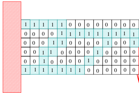
FIG. 1 – Le problème de la plaque-console 2 \times 1 et une représentation “bitarray” (tableau de bits) d’une structure sur un maillage régulier (ici un maillage 13 \times 6 ). Cf. section 3.
