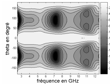
Figure 13 : Diagrammes de rayonnement (niveau en dB), plan H, en fonction de la fréquence, triplaque.
