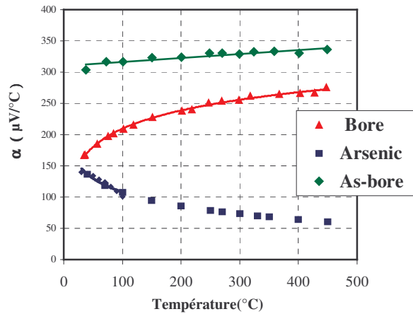
Figure 7 : Evolution du pouvoir thermoélectrique du polysilicium dopé arsenic et bore (dose 10^{16} at/cm 2 ) en fonction de la température
