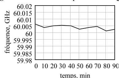
Figure 3 : Instabilité de fréquence de générateur.
