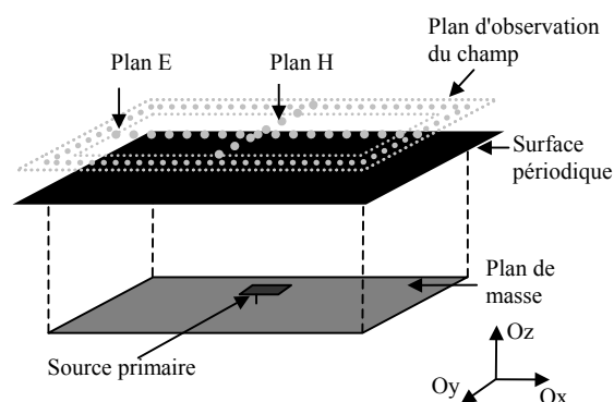
Figure 1: Schéma d'une antenne résonateur BIE
