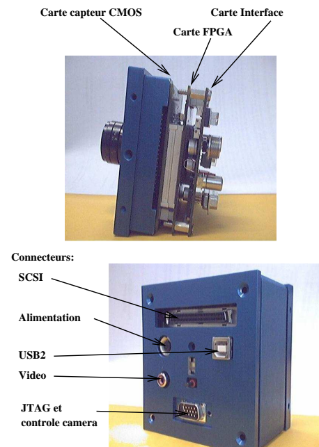
FIG. 1 – Système caméra rapide
