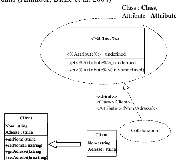
Figure 4 : Spécification d'une transformation de génération des accessors à l'aide d'une collaboration paramétrée
