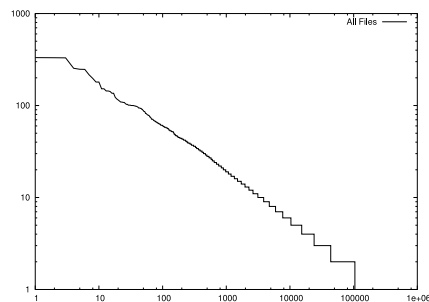
FIG. 11 – Popularités des fichiers en terme de nombre de répliqués dans les caches des nœuds du réseau. Courbe log-log ; en x rang du fichier dans la liste triée selon le nombre de répliqués ; en y le nombre de répliqués du fichier.
