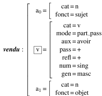
FIG. 1 – Entrée du lexique : forme fléchie vendu correspondant à l'usage transitif du lemme vendre .
