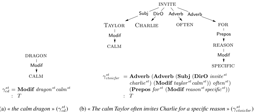
FIGURE 5 – Représentation de SSyntS associées aux expressions « the calm dragon » et « The calm Taylor often invites Charlie for a specific reason » et des termes objets (de \Lambda(\Sigma_{st}) ) associés.
