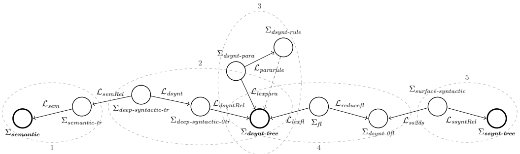
FIGURE 4 – Composition des ACG de l’implémentation de MTT
