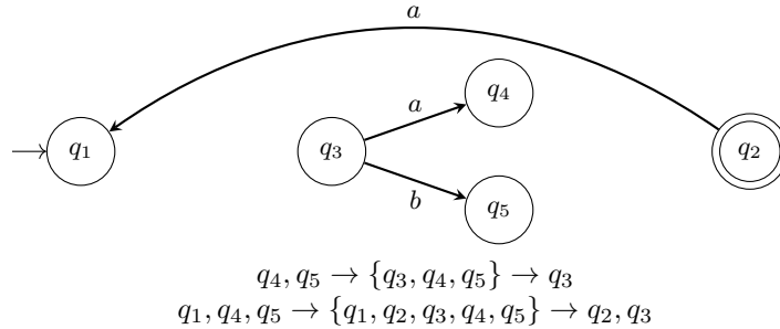
Fig. 5: The input automaton \mathcal{A} .
