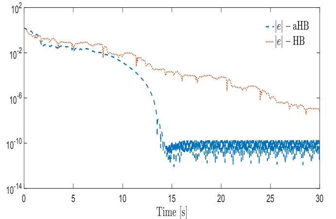
Figure 3. Parameter Identification Error
