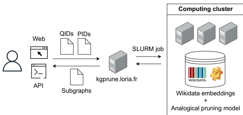
Fig.2. Architecture technique de KGPRUNE. Les utilisateurs peuvent soumettre des tâches d'extraction de sous-graphes via le site Web ou l'API. Ces tâches sont ensuite soumises sous forme de tâches SLURM à notre cluster de calcul.
