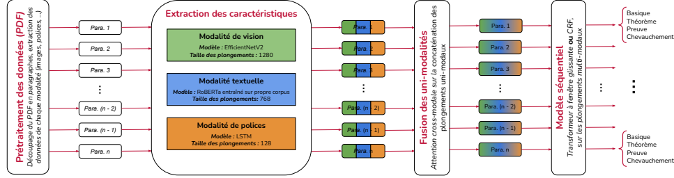
FIG. 1 – Chaîne de traitement pour l'inférence multimodale
