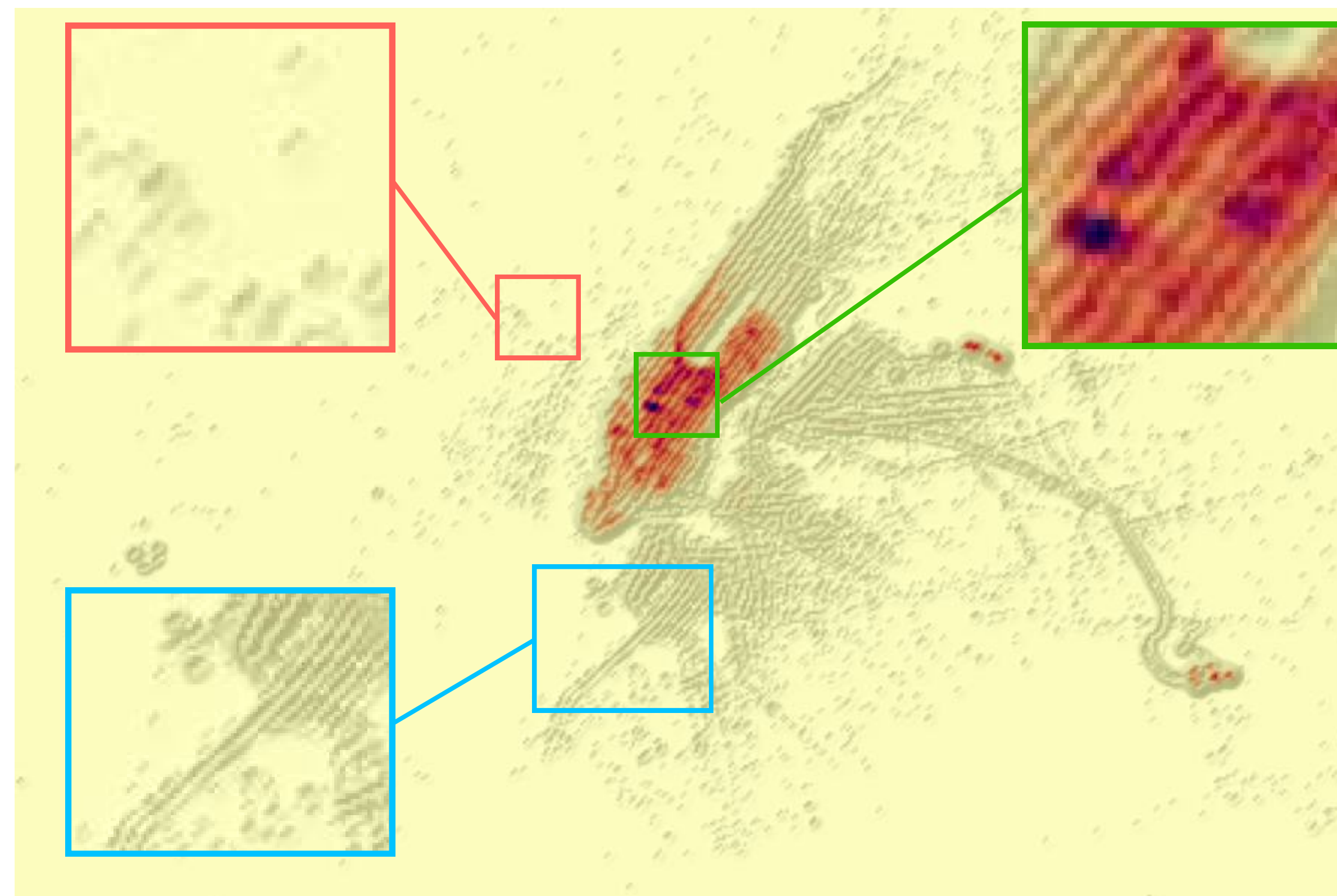
(d) Visualization-driven illuminated density plot
