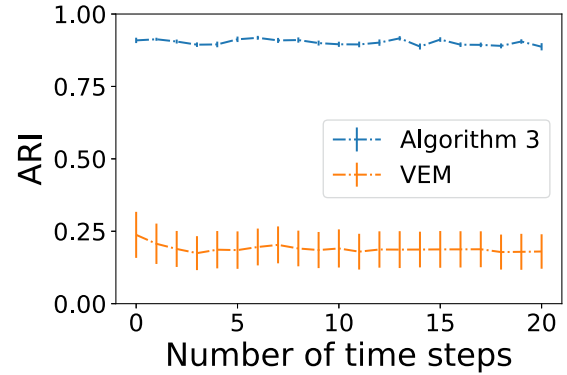
(c) P_{11} = 0.7
