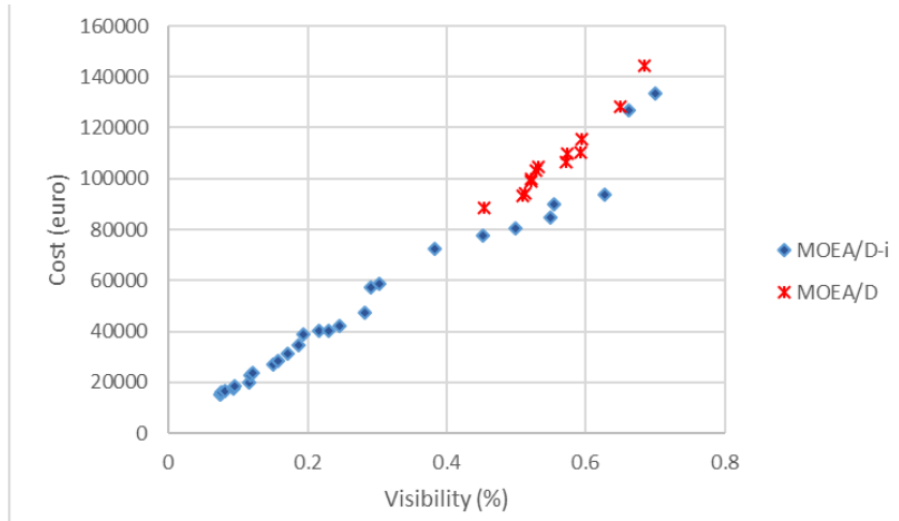
Fig. 3: MOEA/D vs MOEA/D-i
