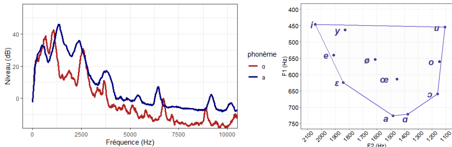
FIGURE 1 : À gauche : spectres comparés de /ɑ/ ( place ) et /ɑ/ ( passe ) ; à droite : trapèze des voyelles orales (F1 et F2 en Hz) produites par un locuteur masculin, archives BnF, 1927.
