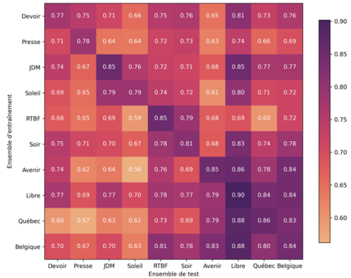
FIGURE 1 & 2 : Exactitudes sur les 10 ensembles de test des 10 modèles CamemBERT (à gauche) et des 10 modèles basés sur des traits (à droite).
