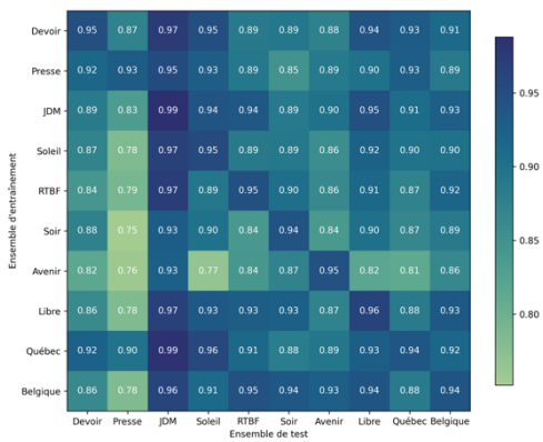
FIGURE 1 & 2 : Exactitudes sur les 10 ensembles de test des 10 modèles CamemBERT (à gauche) et des 10 modèles basés sur des traits (à droite).
