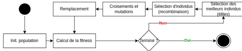
FIG. 1 – Vue simplifiée du fonctionnement d'un algorithme évolutionnaire.
