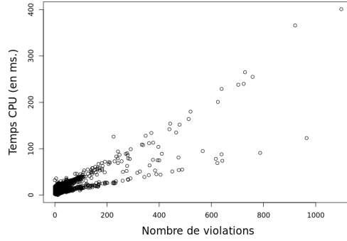
FIG. 5 – Temps d'exécution CPU des formes SHACL découvertes en fonction du nombre de violations observées.
