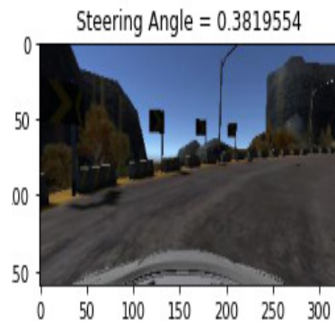
Fig. 22. True SA = 0.381
