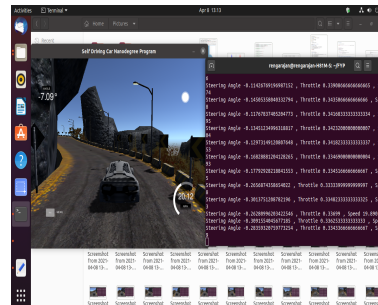
Fig. 19. Predicted SA = -0.283
