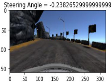
Fig. 18. True SA = -0.238
