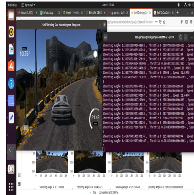
Fig. 23. Predicted SA = 0.430
