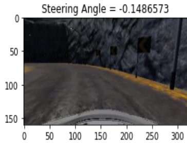
Fig. 16. True SA = -0.148
