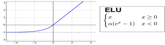
Fig. 10.ELU Function
