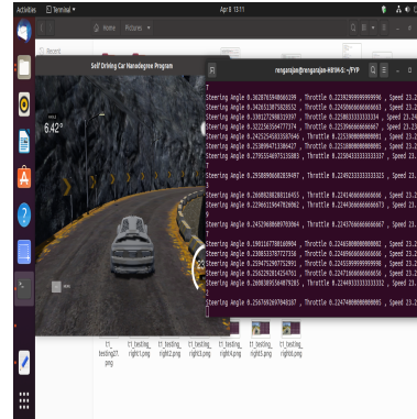
Fig. 21. Predicted SA = 0.256
