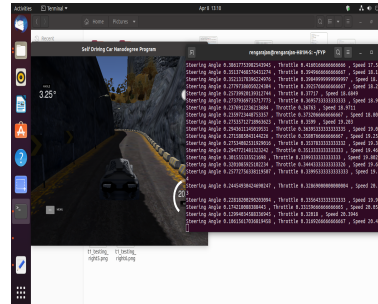
Fig. 17. Predicted SA = -0.106
