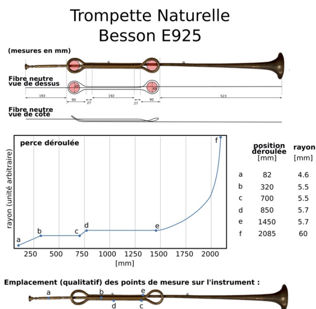
FIGURE 13 – Plan de la copie acoustique de la trompette E.0925.
