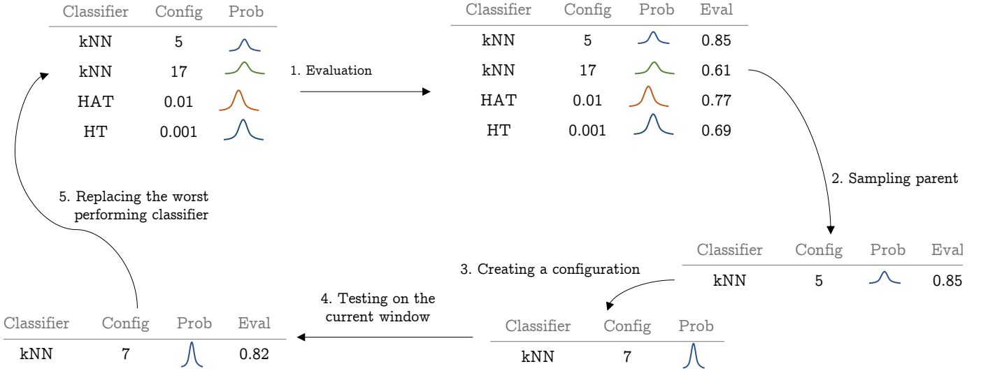
Fig. 1: AutoClass.
