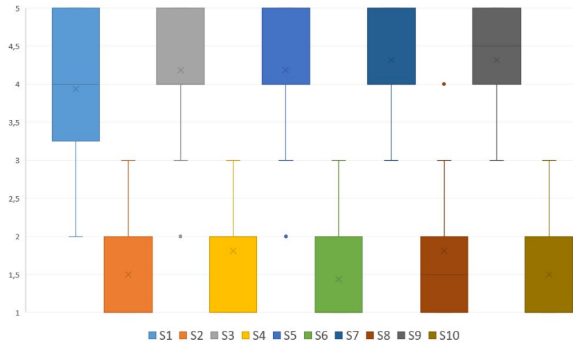
Fig. 6. SUS scores
