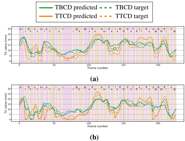
Figure 3: TBCD and TTCD trajectories for the utterance "En écoutant la flûte, le chevreau mangea la robe à froufrous de Maurine". Authorized reproduction from [25].
