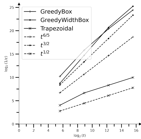
(d) Error rate in 2-norm on g^t
