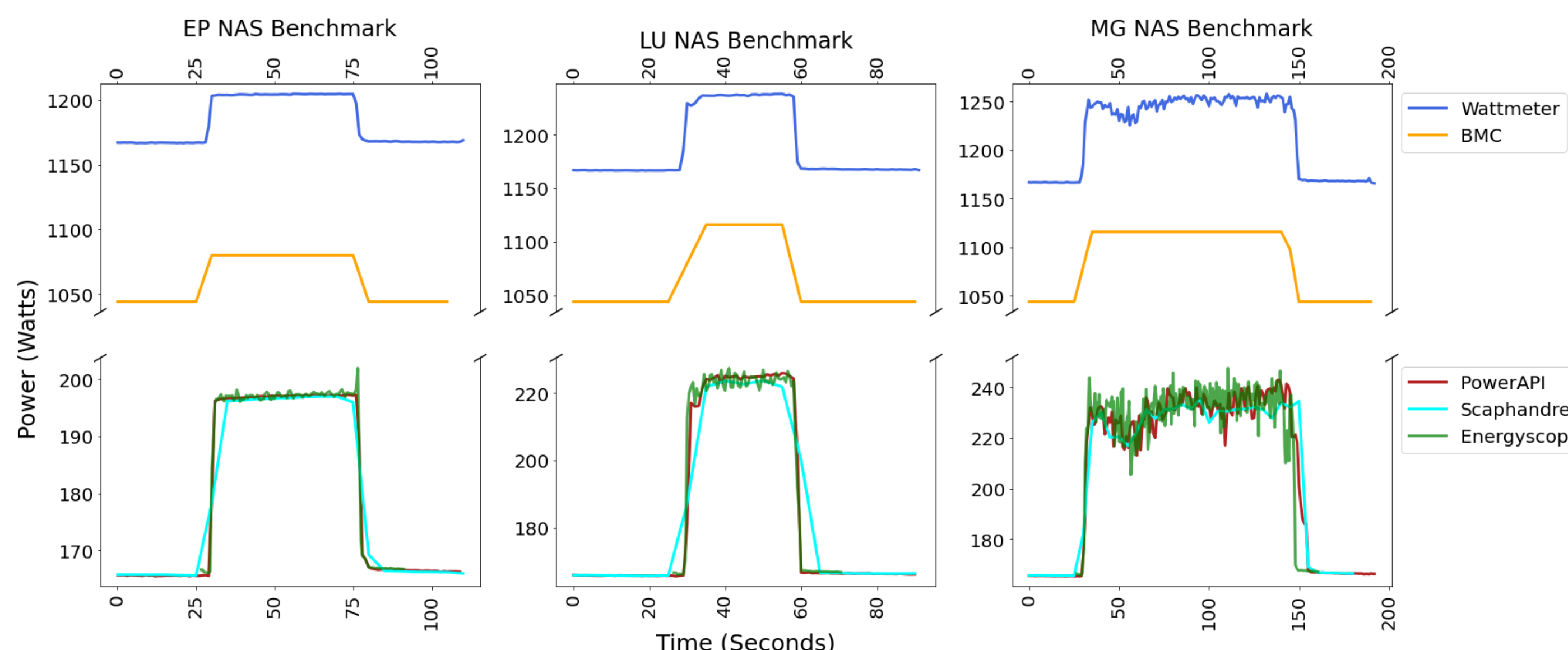
Figure 2. Profilage de puissance
