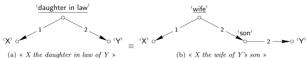
FIGURE 13 – Illustration de l'équivalence de deux graphes pour la paraphrase sémantique
