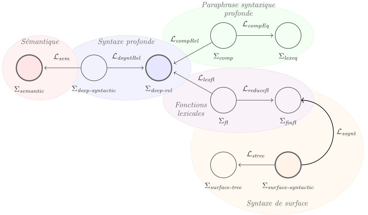
FIGURE 10 – Aperçu de l'architecture des ACGs
