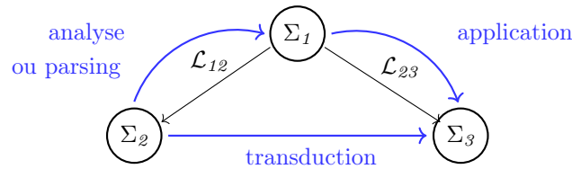
FIGURE 1 – Schéma illustratif d'un ensemble d'ACGs
