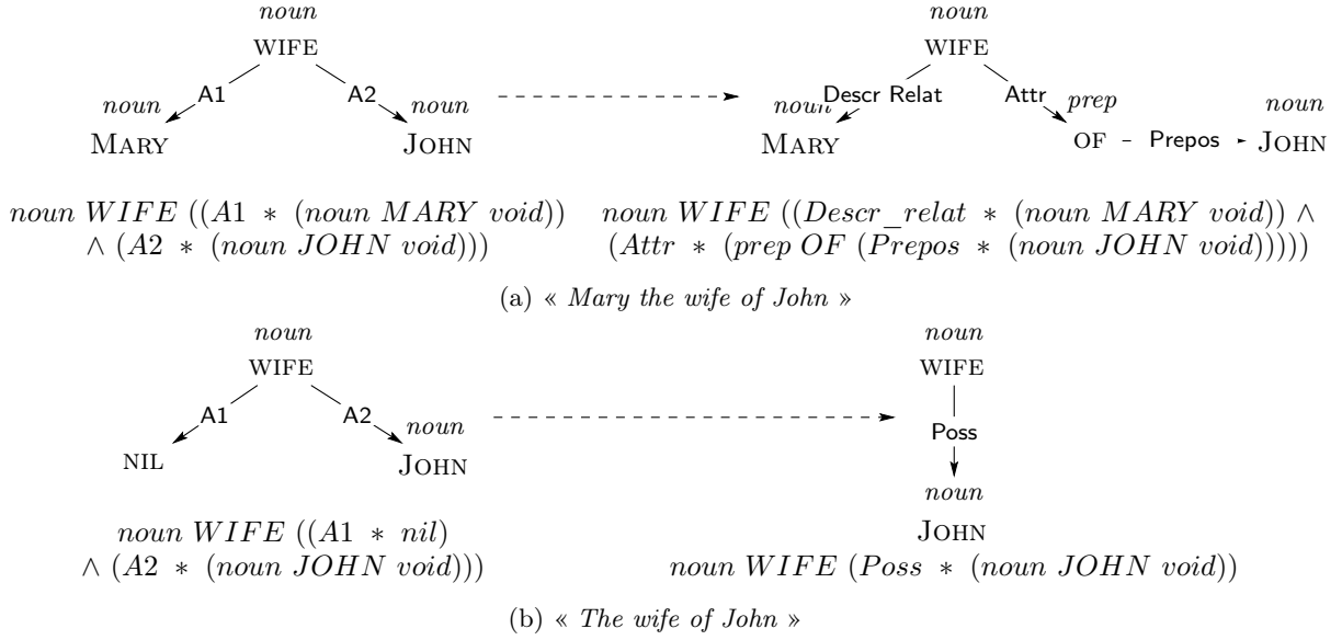
FIGURE 22 – Illustration des arguments optionnellement exprimables dans les représentations en syntaxe profonde (à gauche) dans \Lambda(\Sigma_{deep-rel}) (ou \Lambda(\Sigma_{finfl}) ) et en syntaxe de surface (à droite) dans \Lambda(\Sigma_{surface-tree}) , accompagnés des \lambda -termes correspondant
