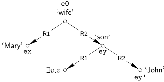
(a) Représentation du graphe sémantique de « Mary, the wife of John's son » dans \Sigma_{semantic} , dont le \lambda -terme correspondant est : \lambda e0. \exists ex ey. (wife\ e0) \wedge (R1\ e0\ ex) \wedge (R2\ e0\ ey) \wedge (mary\ ex) \wedge (\exists ex'\ ey'. (son\ ey) \wedge (R1\ ey\ ex') \wedge (R2\ ey\ ey') \wedge (\exists v.v\ ex') \wedge (john\ ey'))
