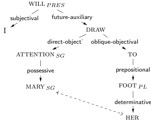
FIGURE 9 – Exemple de structure syntaxique de surface (Mel’čuk et al. 2012, p109) pour la phrase « I will draw Mary’s attention to her feet. ».
