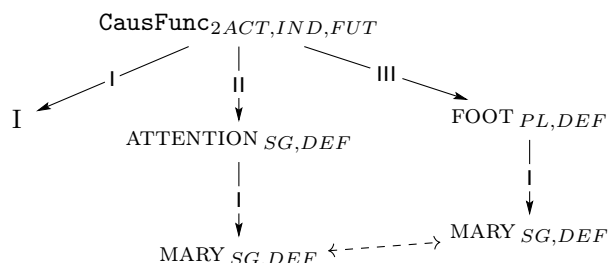
FIGURE 7 – Exemple de structure syntaxique profonde (Mel'čuk et al. 2012, p107) pour la phrase « I will draw Mary's attention to her feet. » (la flèche en pointillés fait partie de la structure anaphorique cf. annexe A).
