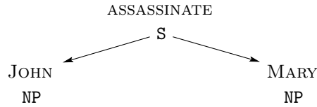
FIGURE 32 – Illustration de « John assassinate Mary » dans \Lambda(\Sigma_{tree})
