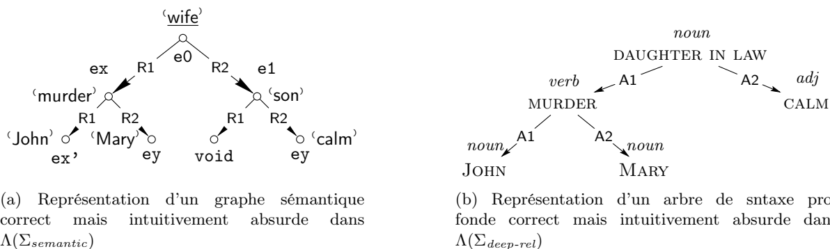
FIGURE 23 – Représentation dans \Lambda(\Sigma_{semantic}) et \Lambda(\Sigma_{deep-rel}) d'une même "phrase" qui n'aura pas de suite dans la génération vers la syntaxe de surface
