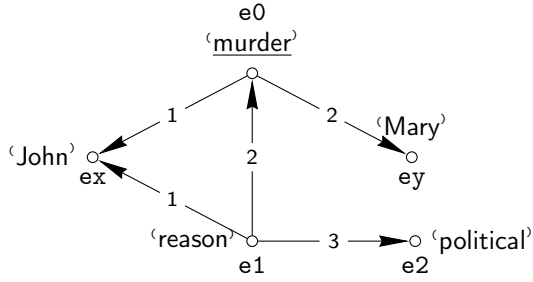
(a) Illustration de la représentation de la phrase « John assassinate Mary. » dans \Sigma_{semantic} , dont le \lambda -terme correspondant est : \lambda e0. (\exists ex ey ez. (murder\ e0) \wedge (R1\ e0\ ex) \wedge (R2\ e0\ ey) \wedge (john\ ex) \wedge (mary\ ey) \wedge (\exists e1\ e2. (reason\ e1) \wedge (R1\ e1\ ex) \wedge (R2\ e1\ e0) \wedge (R3\ e1\ e2) \wedge (politics\ e2)))
