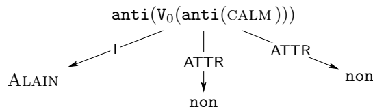
FIGURE 19 – arbre de syntaxe profonde ayant une structure erronée
