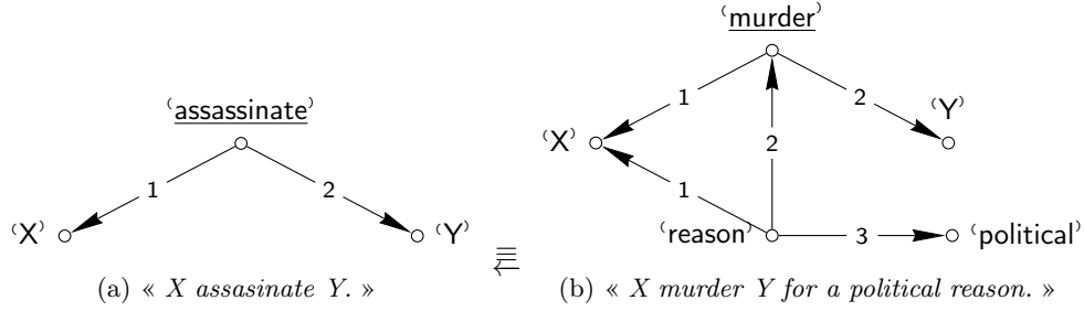
FIGURE 14 – Illustration de l'équivalence de deux graphes pour la paraphrase sémantique lorsqu'un sens de paraphrase est préféré
