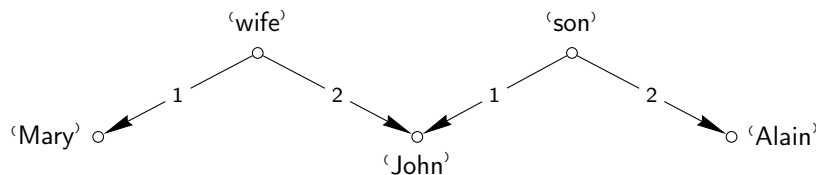
FIGURE 15 – « Graphe sémantique irréalizable »
