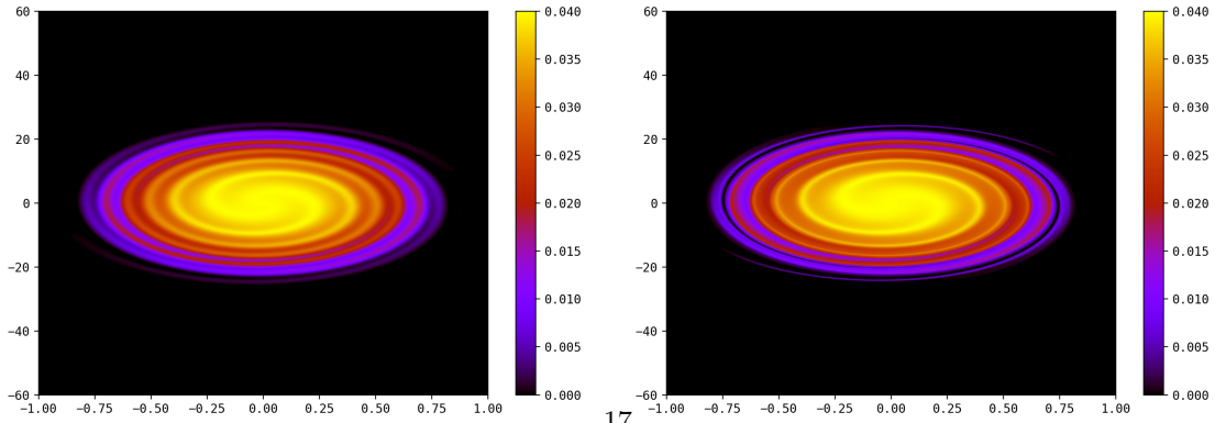
(d) Electron distribution function
