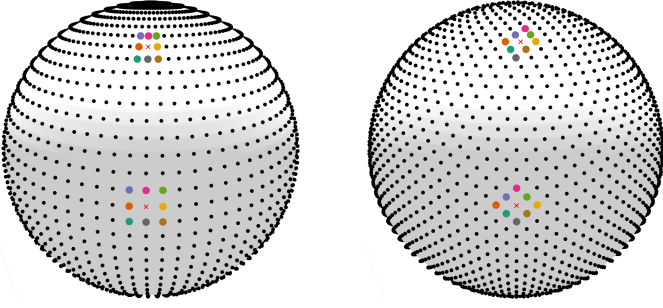
FIGURE 3 – Représentation du noyau de convolution à différents endroits de la sphère pour deux échantillonnages : équirectangulaire à gauche, et HEALPix à droite.
