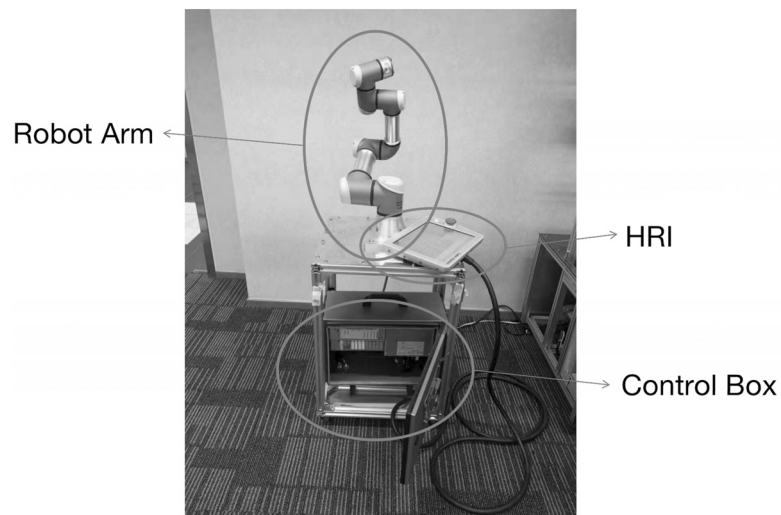
Figure 1. Universal Robot (Version 3.5.1.10661)
