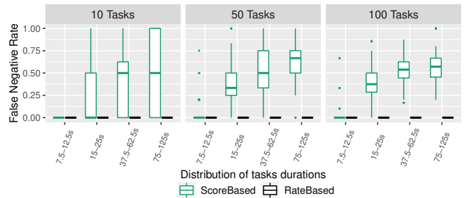
(d) SKEWEDSTARTS-WITHLATENCY
