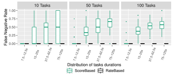
(d) SKEWEDSTARTS-WITHLATENCY
