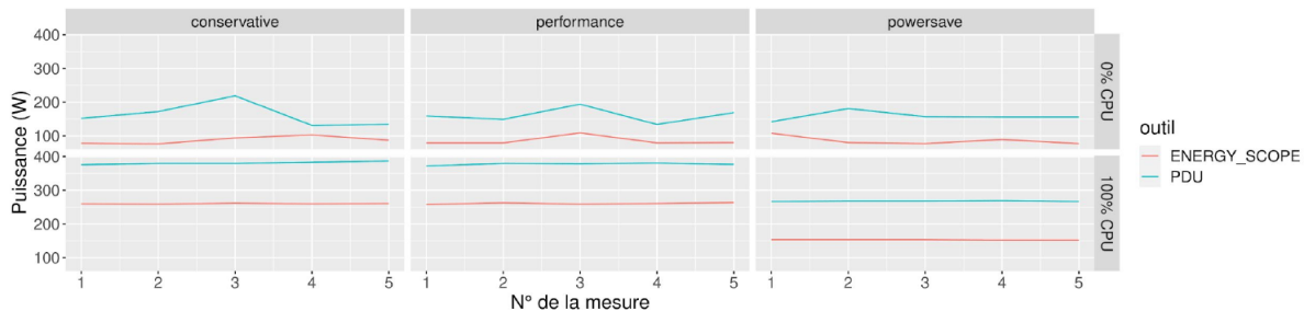
FIGURE 8 – Comparaison energy_scope / PDU sur diablo04 en fonction de l'utilisation du CPU et du governor
